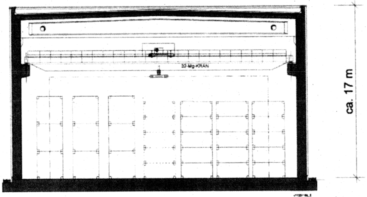
Abbildung 5.1.2-2: Querschnitt des LAW 2 (IA-2, Abb. 3, mit Beispielbelegung 2)
